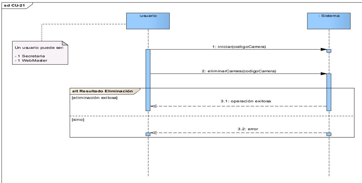
Figura C. 21 Diagrama de Secuencia Caso de uso "Eliminar carrera"
