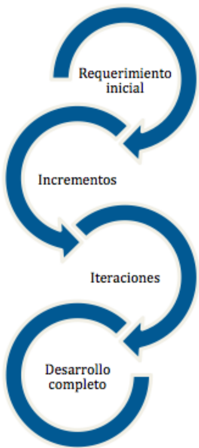
Figura 7. Metodología iterativa [5]
