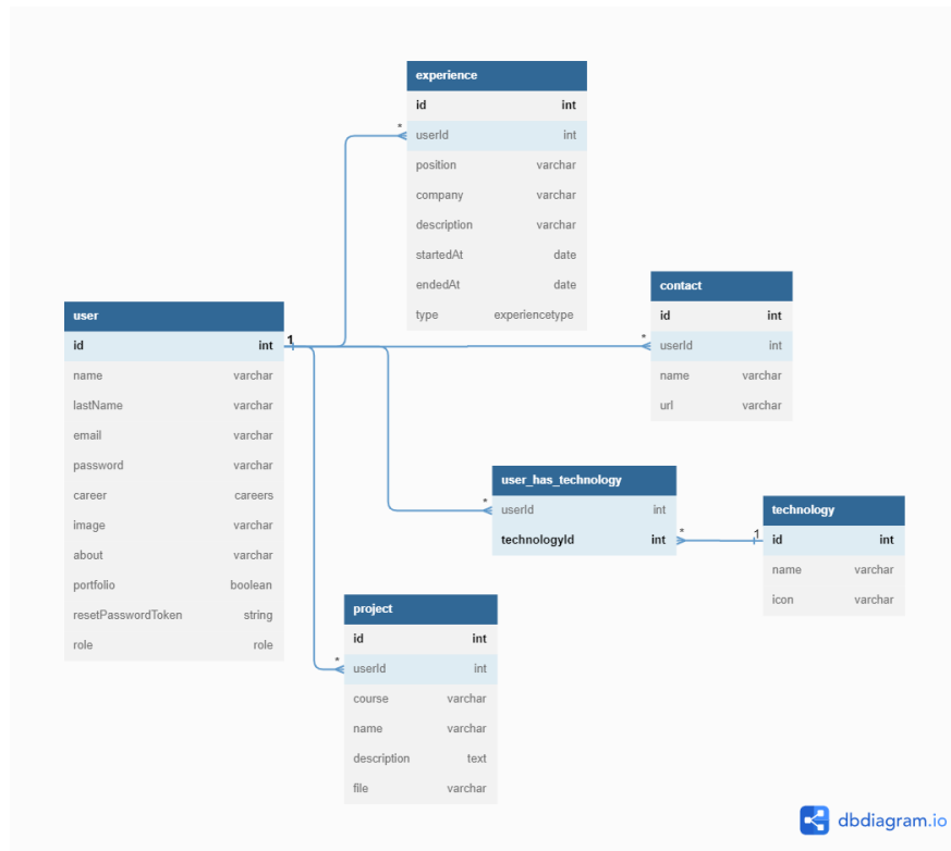
Figura 14. Modelo Relacional
