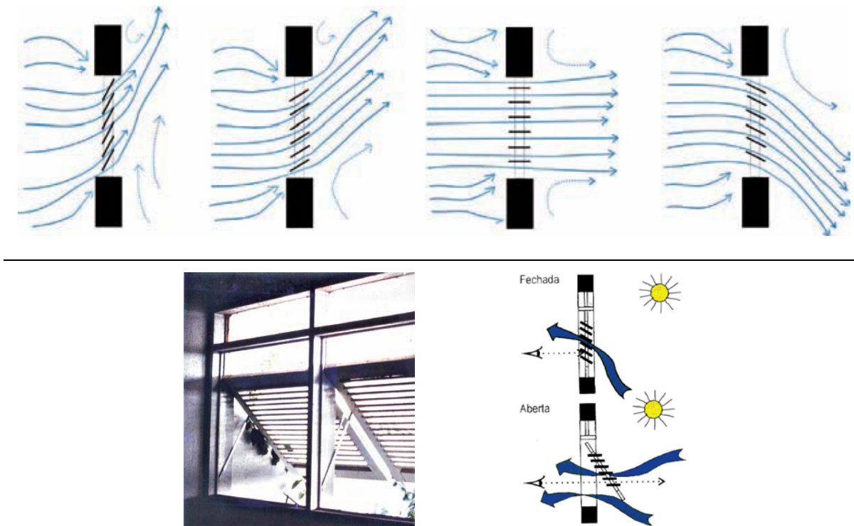
Figura 22: Venezianas móveis para a regulação do fluxo de ar
