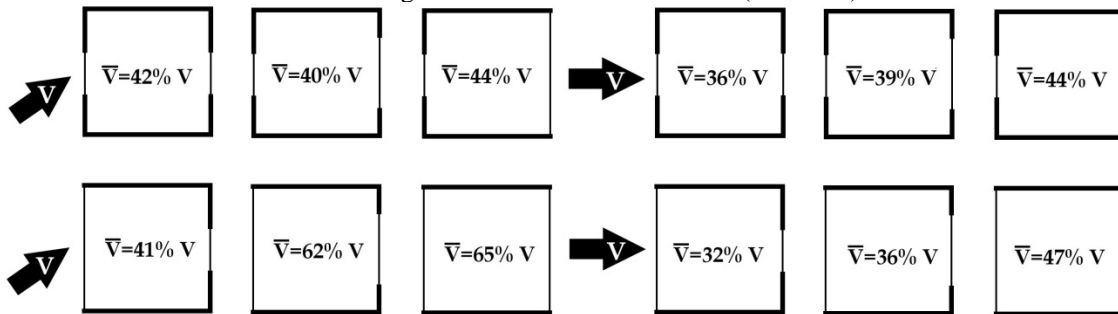
Figura 20: Velocidade média interna no ambiente em relação às aberturas de entrada e saída do ar para dois ângulos diferentes de incidência (45° e 90°)
