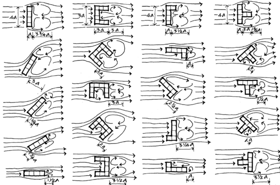
Figura 18: Comportamento do fluxo de ar em diversificadas soluções em plantas baixas
