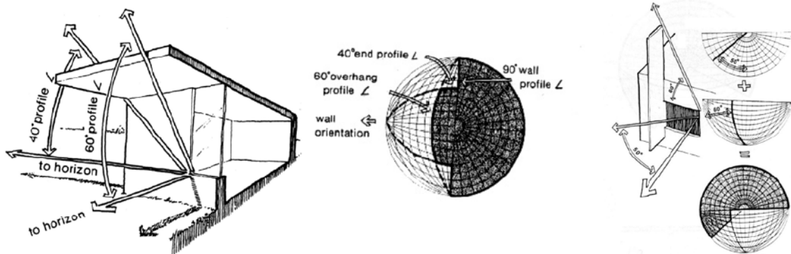
Figura 13: Fatores interferentes na definição dos dispositivos de sombra
