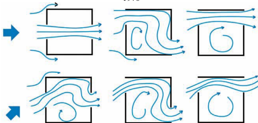
Figura 21: Distribuição do fluxo de vento de acordo com a localização das aberturas para a orientação de incidência do vento perpendicular e oblíqua à abertura. Trabalho desenvolvido por Baruch Givoni em 1976
