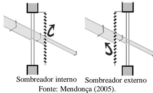
Figura 11: Posicionamento dos dispositivos de sombra
