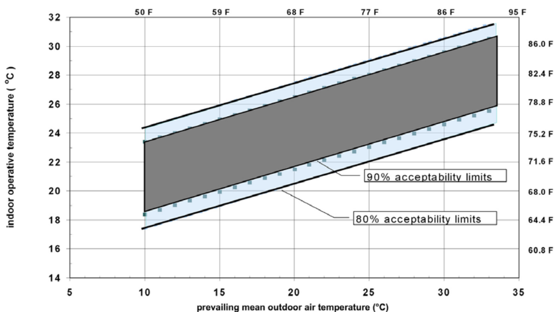
Gráfico 3: Modelo de conforto adaptativo
