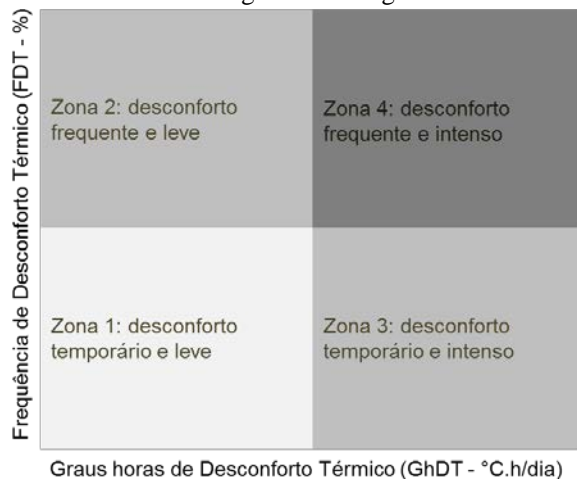
Figura 31: Diagrama de flutuabilidade dos indicadores FDT e GhDT
