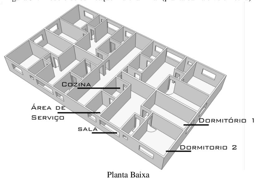
Figura 32: Modelo de edificação multifamiliar (planta baixa e volumetria)
