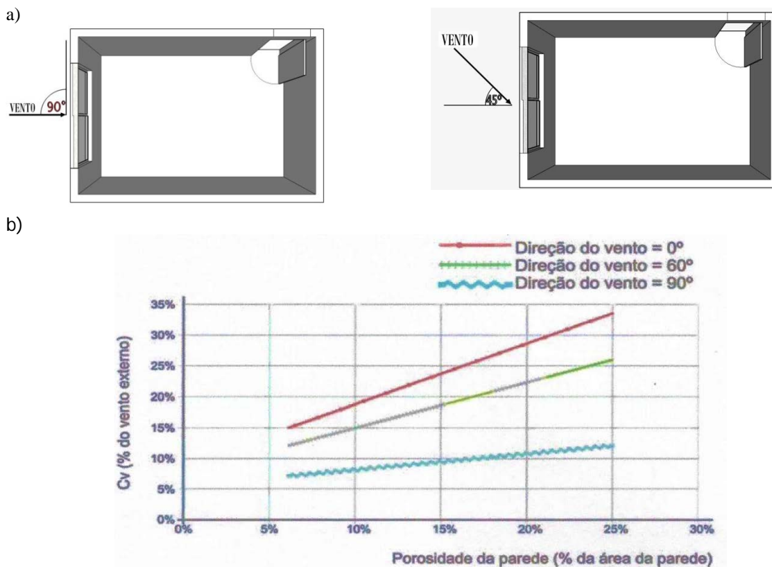
Figura 15: a) Posicionamento das aberturas e b) Percentual de vento em relação à porosidade da parede
