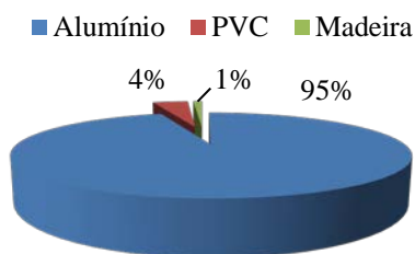
Gráfico 9: Tipos de materiais observados nos modelos de janelas
