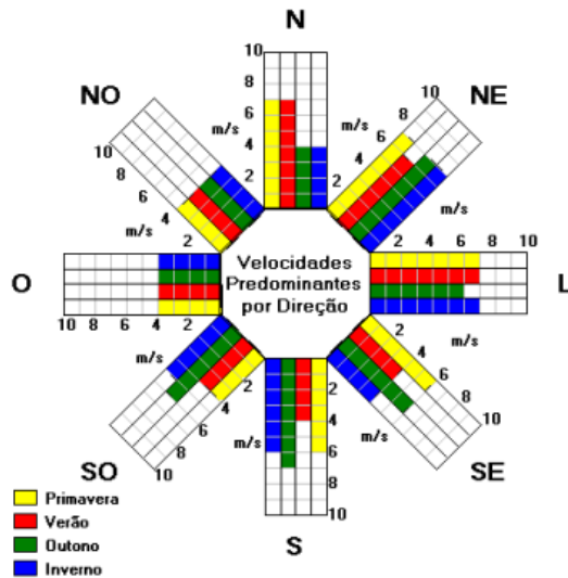
Gráfico 5: Frequência de ocorrência e direção dos ventos, para a cidade de Vitória. a) Direção e velocidade do vento; b) Frequência da velocidade do vento
