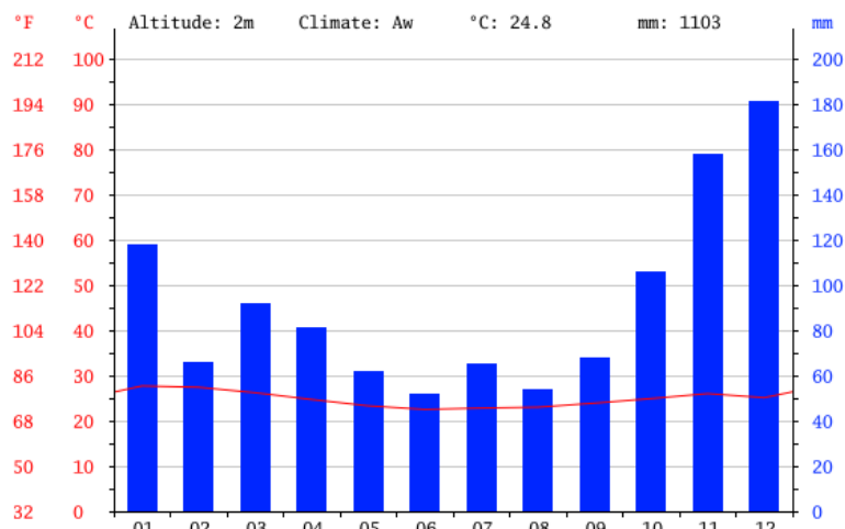
Gráfico 6: Variações da temperatura externa em Vitória
