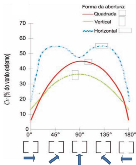
Figura 14: Flutuações do rendimento médio da incidência do vento para três formatos de abertura
