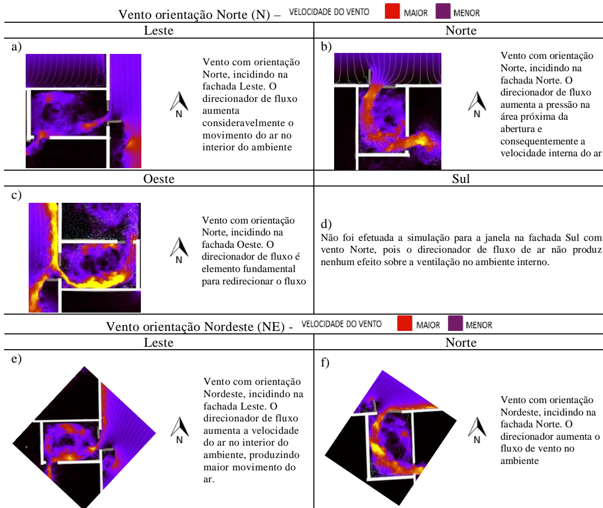
Figura 34: Posicionamento da abertura para cada orientação utilizando as simulações com o software Wind Tunnel-Pro
