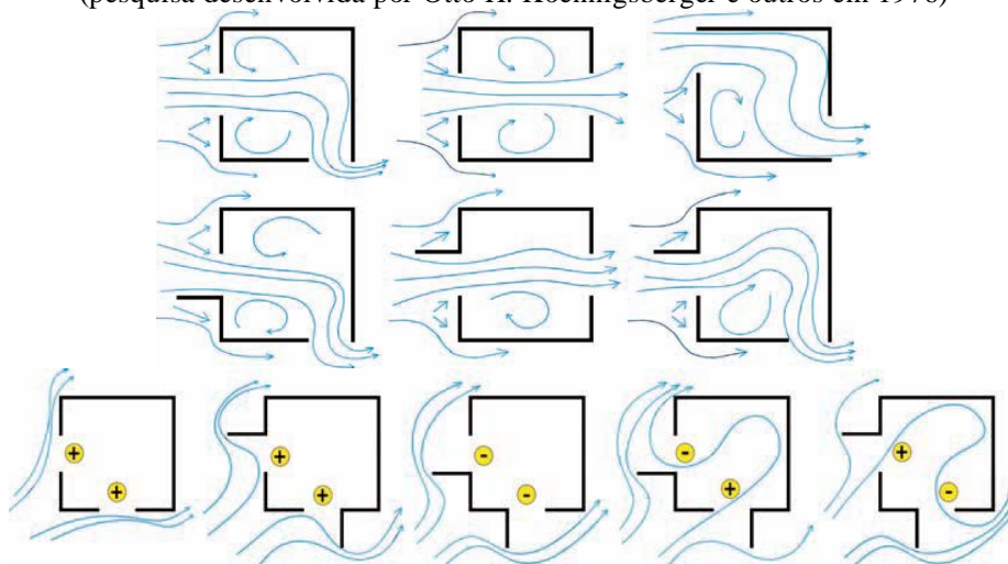
Figura 23: Interferência dos componentes verticais na distribuição do fluxo de ar no interior dos ambientes (pesquisa desenvolvida por Otto H. Koennigsberger e outros em 1976)
