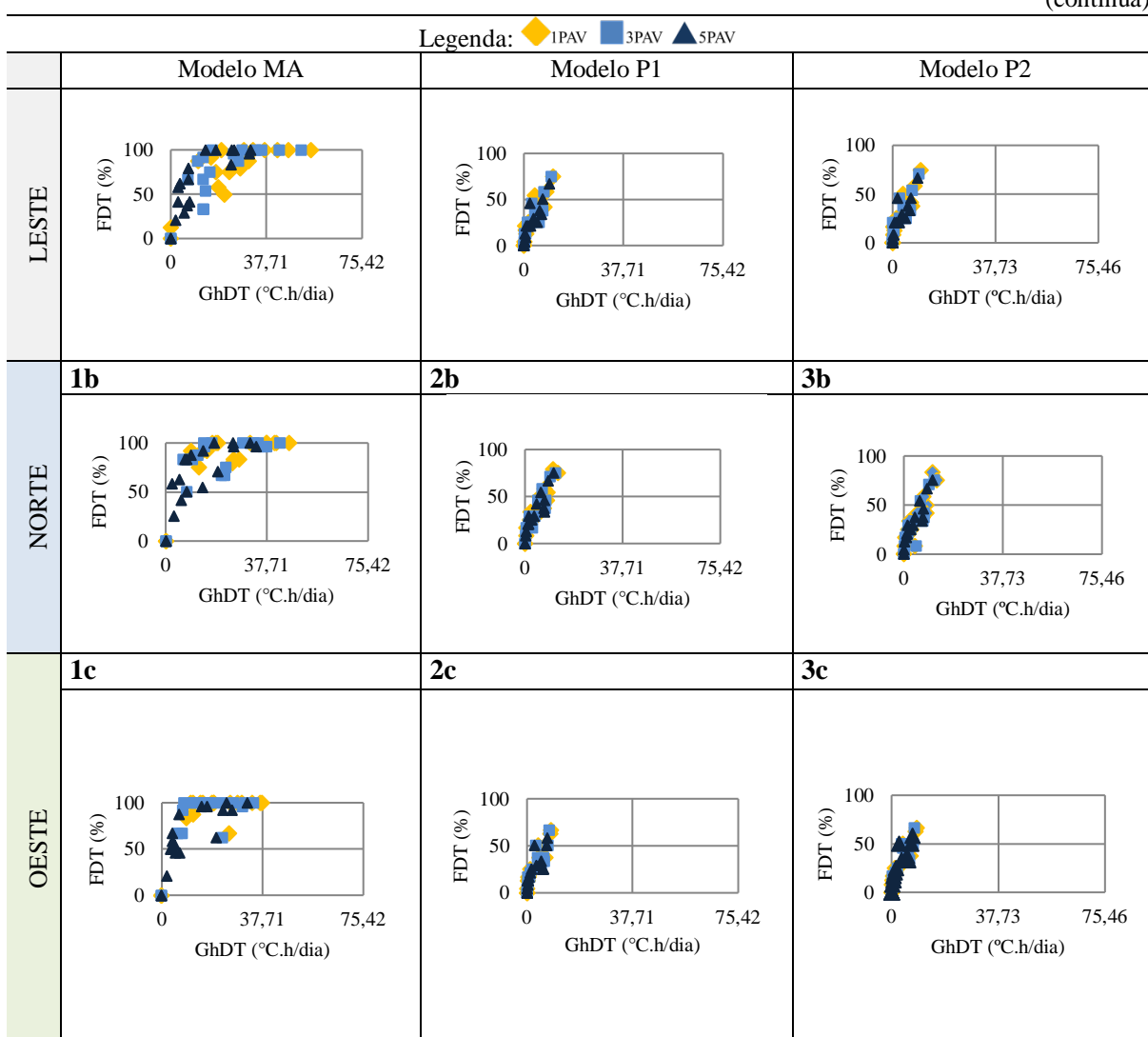
Gráfico 18: Diagramas de fluatibilidade dos três modelos de janela para a primavera
