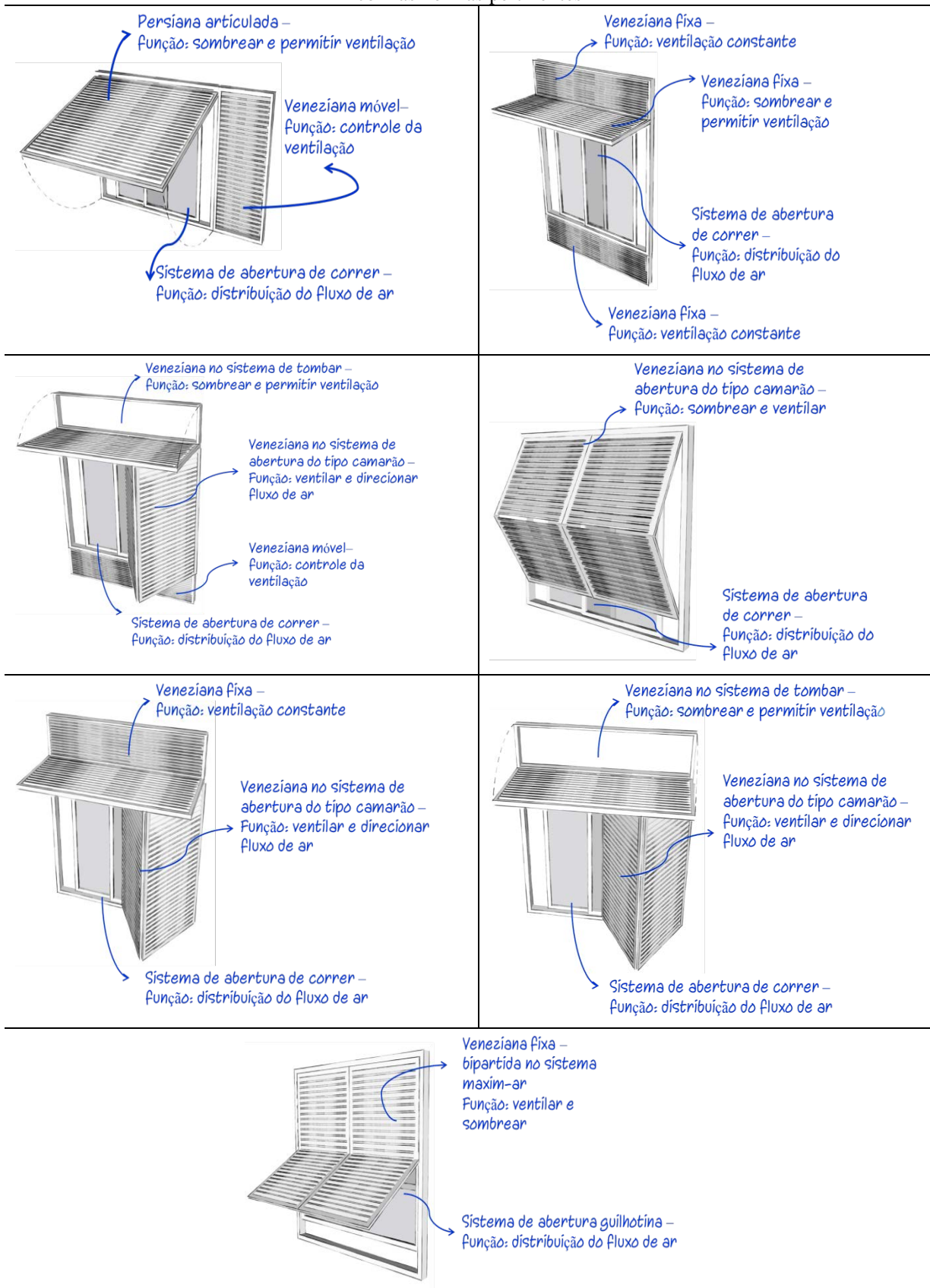
Figura 35: Desenhos adicionais de janelas considerando os resultados obtidos nas simulações e de acordo com as normas pertinentes
