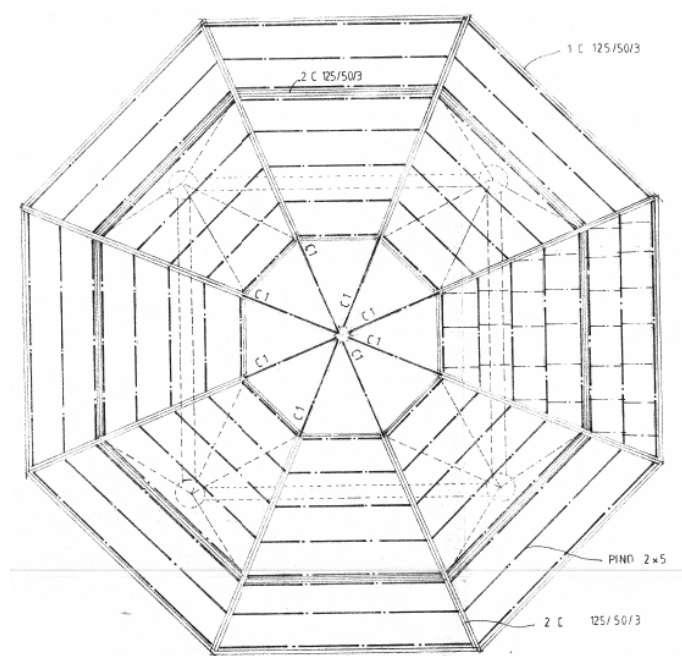
Plano estructura de techumbre
