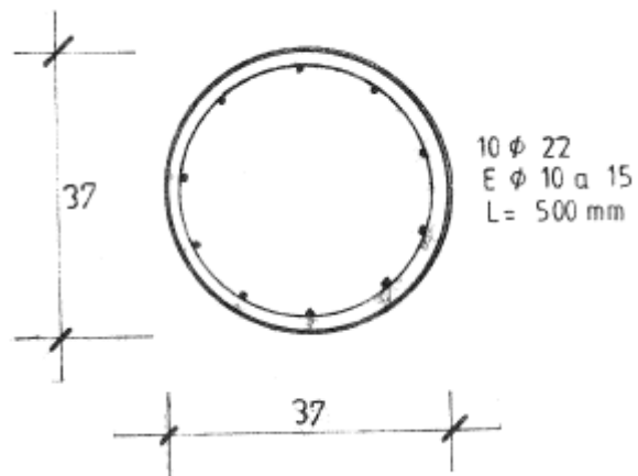
Detalle pilar pérgola de las flores. Plaza sargento Aldea Chillan.
