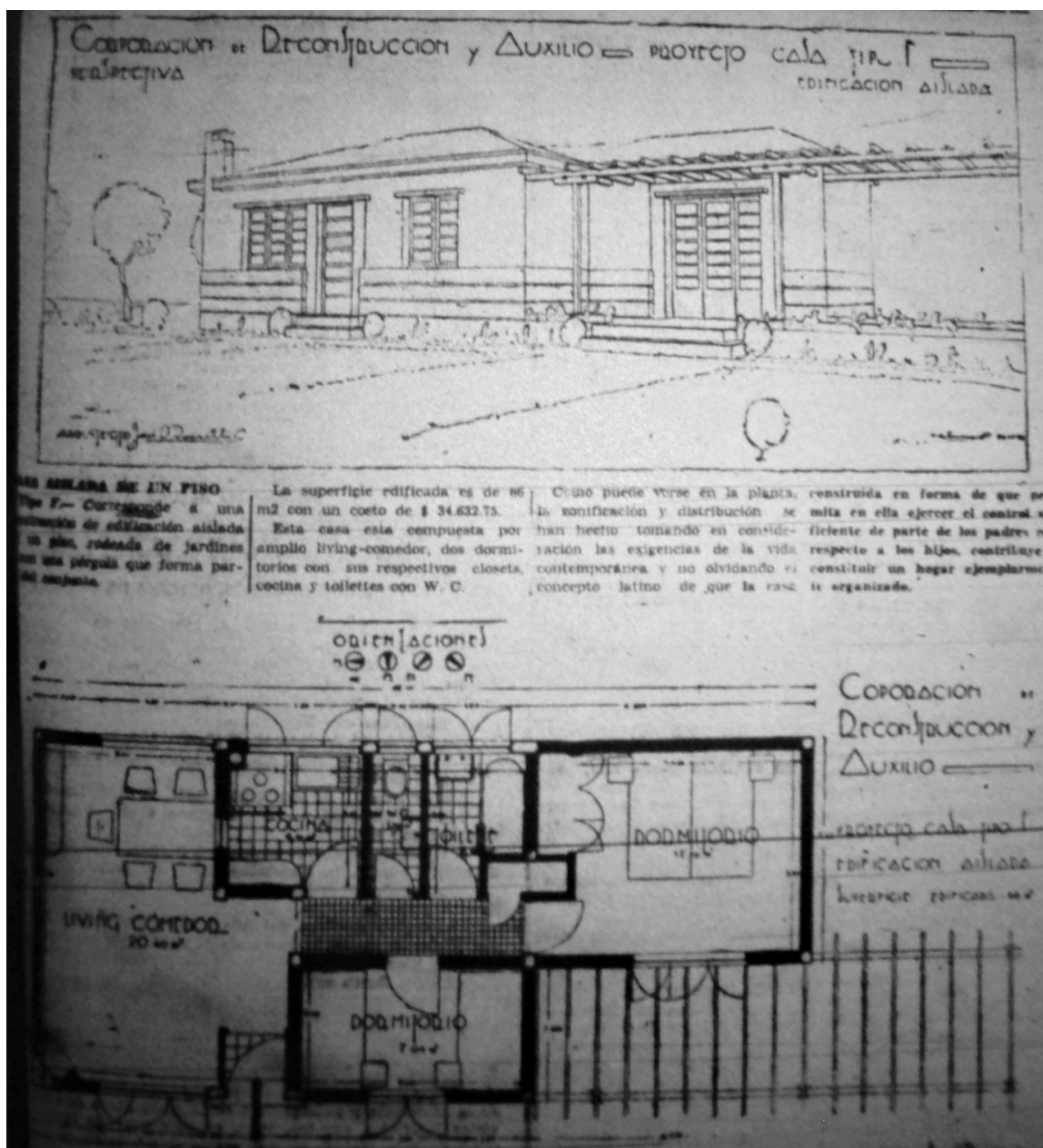
Plano de casas tipo. Casa Tipo F Corporación de Reconstrucción y Auxilio Fuente: La Discusión, 14 de enero de 1940
